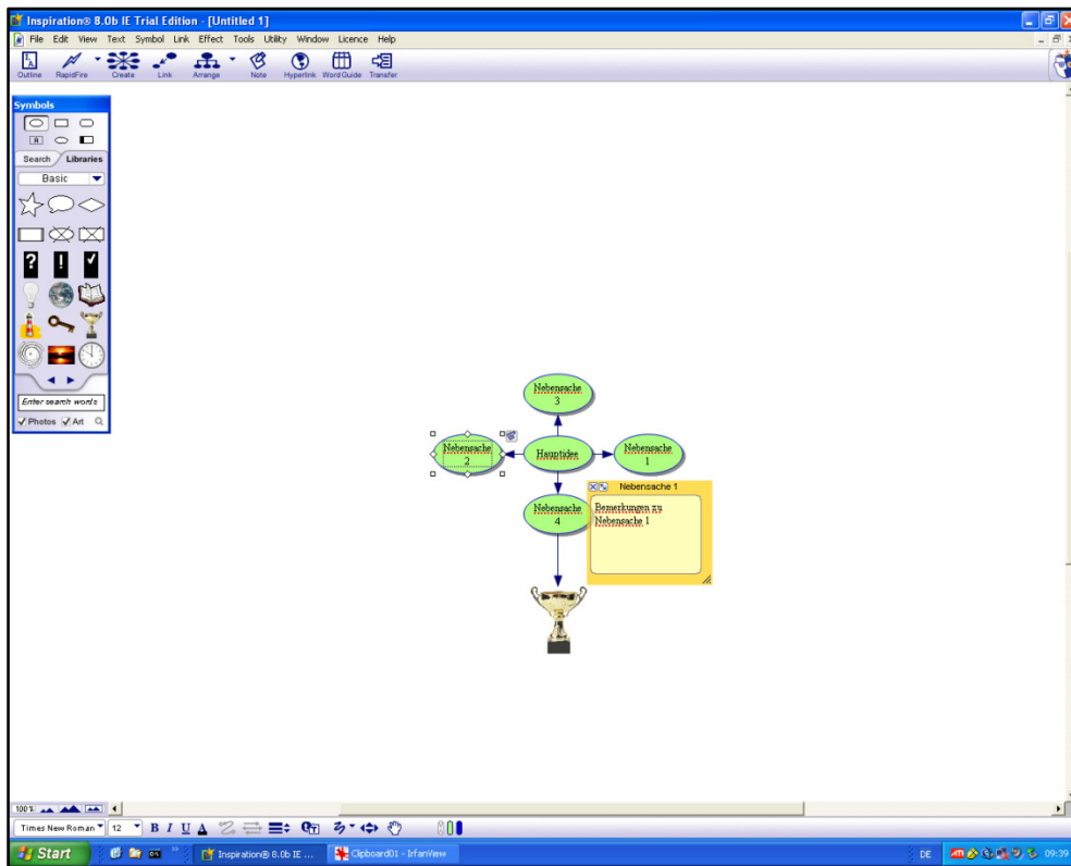
Abb. 1: Diagramm-Ansicht
