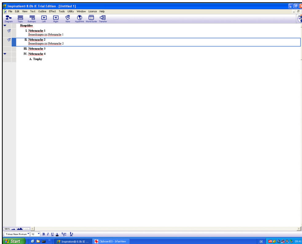
Abb. 3: Outline-Ansicht
