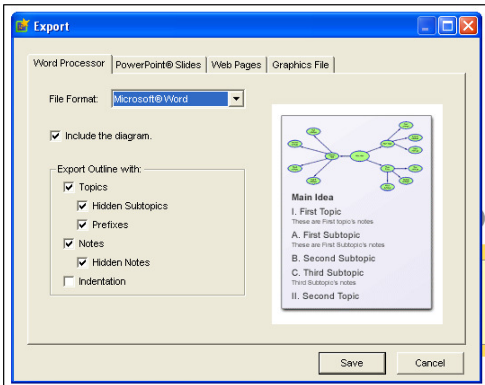
Abb. 4: Exportfunktionen
